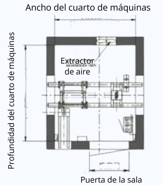
Plano del cuarto de máquinas
