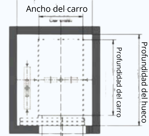
Plano de hueco de ascensor con apertura lateral
