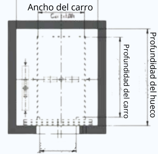
Plano del hueco del ascensor en el medio
